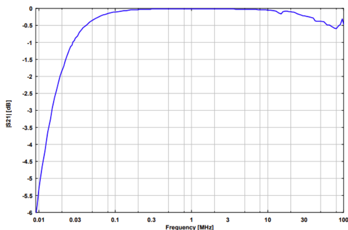
EUT 到 BNC 传输损耗
