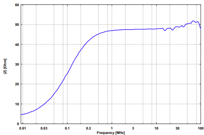
EUT 端阻抗曲线
