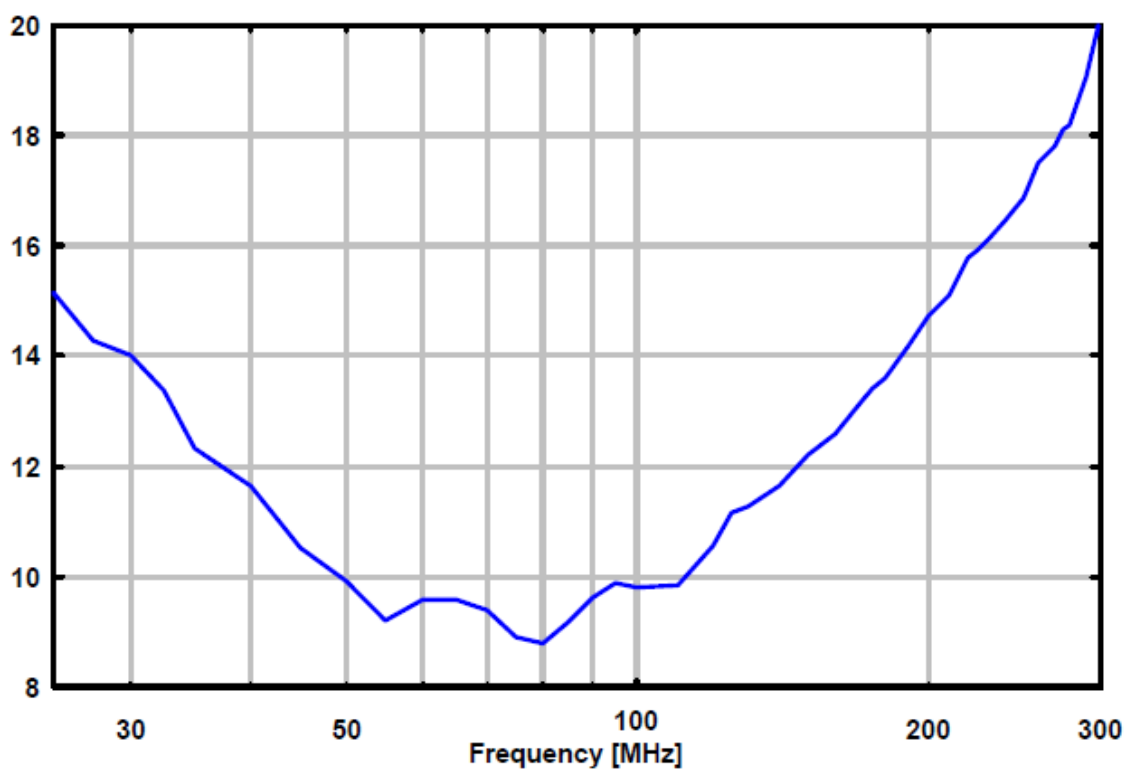
天线因子 (dB/m)
