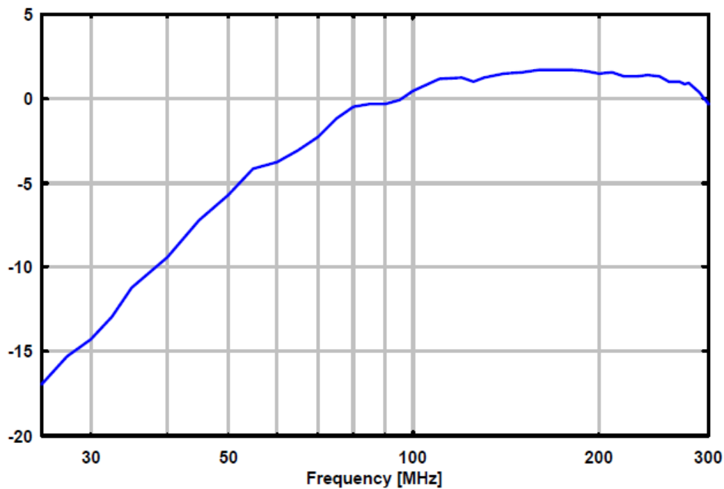
天线增益 (dBi)
